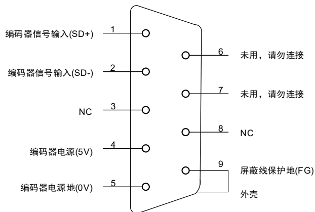
驱动器X2插头（绝对值编码器）
