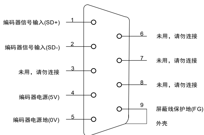
驱动器X2插头（增量式编码器）
