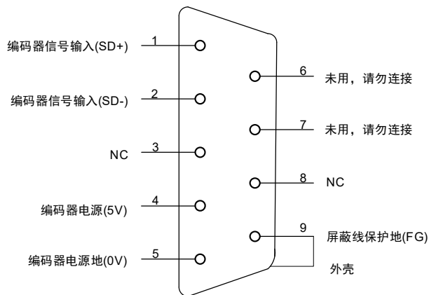
驱动器X2插头（绝对值串行通信编码器）
