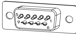
X3B 插头焊针分布图
