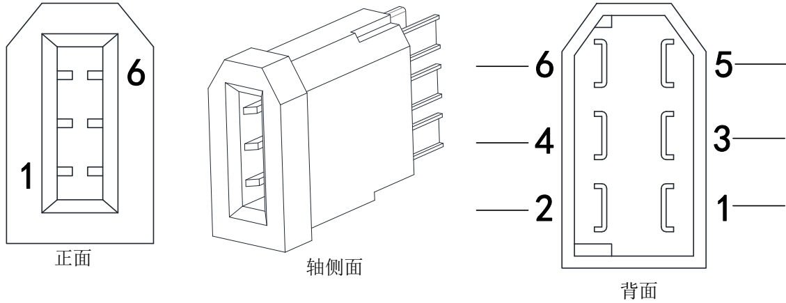
CN2-A、CN2-B接头芯子针脚图 驱动器 CN2-A、CN2-B 插头
