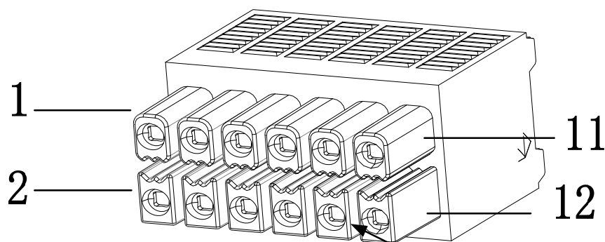
CN1-A/B插头尾端示意图，接线时仔细注意线孔序号 根据尾端的形状来判断孔序号
