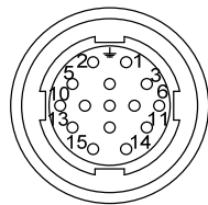
110/130/180电机编码器插头
