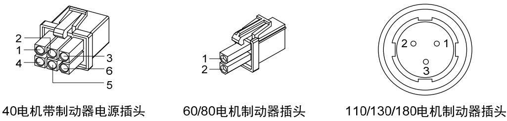
40 电机带制动器电源接线：
