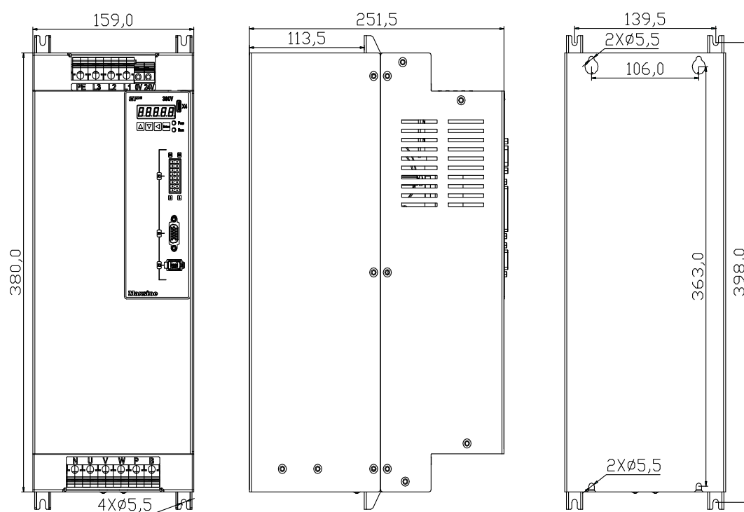
TH110、TH150 安装尺寸图
