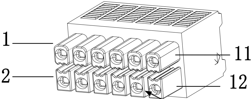
CN1-A/B插头尾端示意图，接线时仔细注意线孔序号
