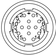
110/130/180电机编码器插头
