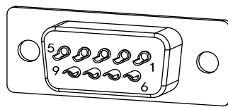
X3B 插头焊针分布图
