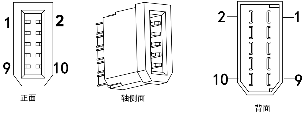
X2接头芯子针脚图
