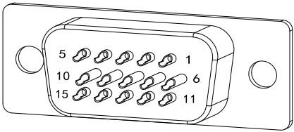
X3A 插头焊针分布图
