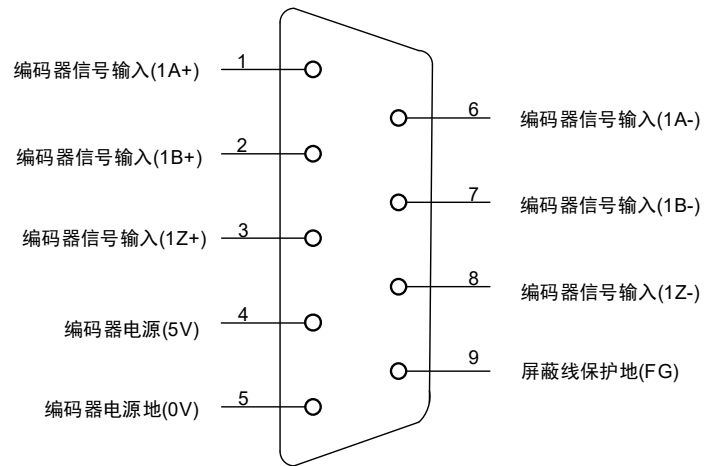
驱动器X3B插头
